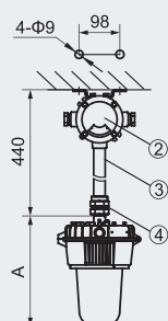
G: pendant pole type
