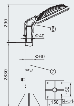
L: pole type
