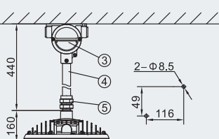
G: pendant pole type
